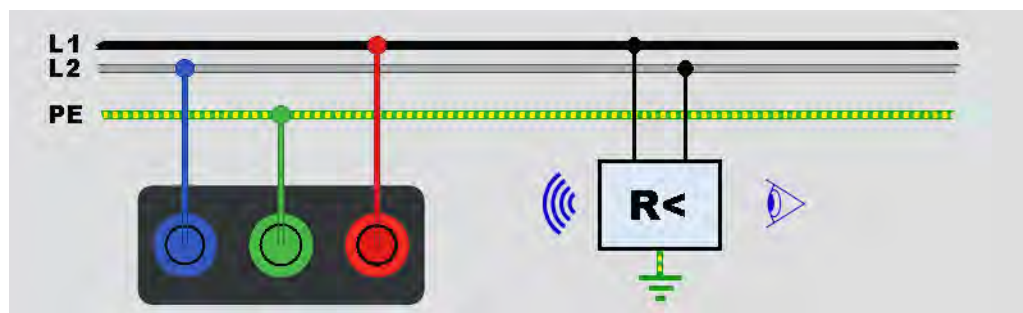
Abbildung 23. IMD-Prüfung Nr. 1
