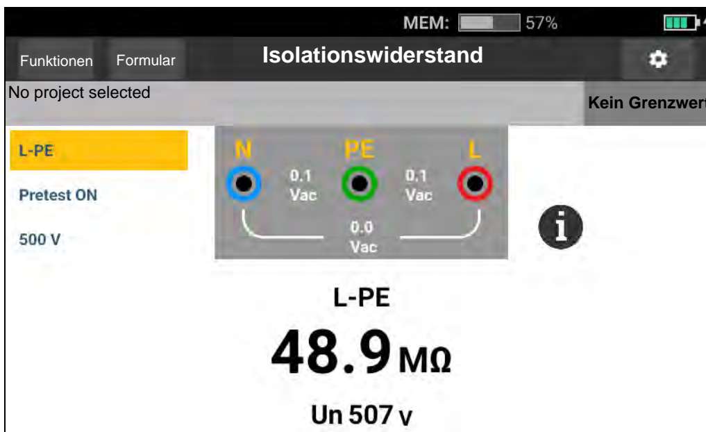
Abbildung 9. Isolationswiderstandsmessbildschirm
