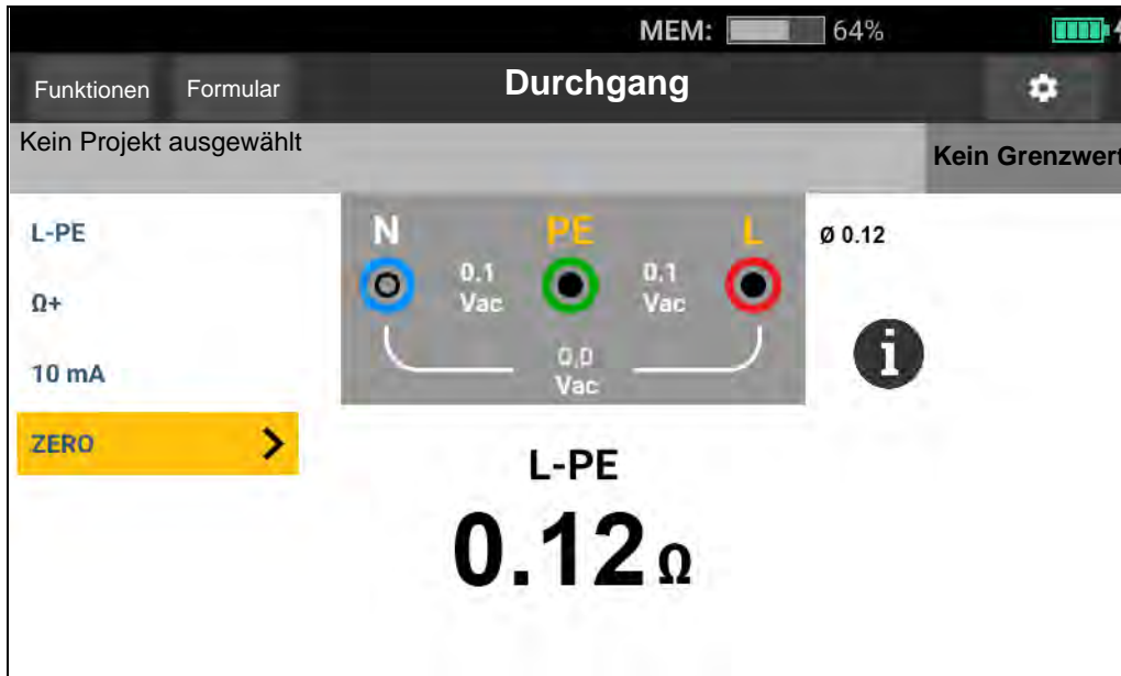
Abbildung 10. Durchgangsprüfungs-Bildschirm
